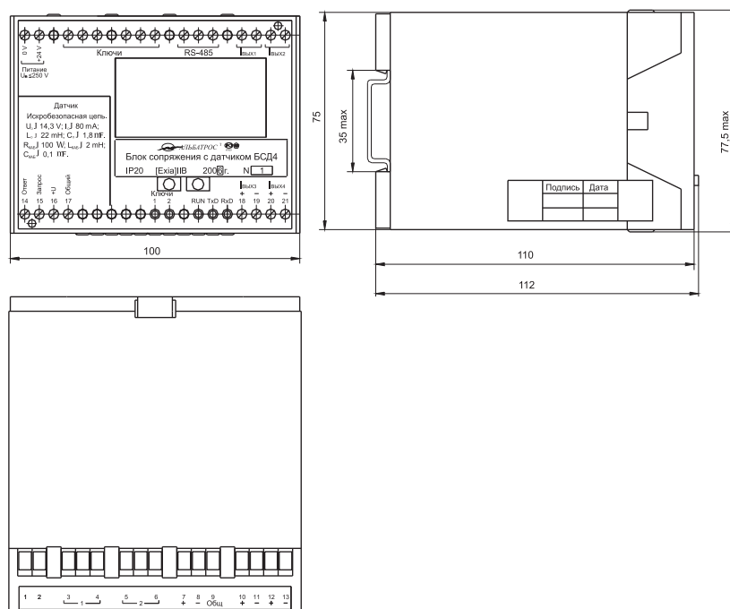
Рисунок II.5.1 – Габаритные размеры блока БСД4
